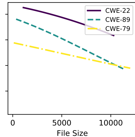
gpt-4o
