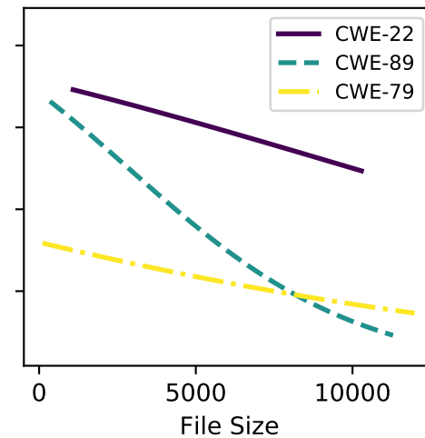
gpt-3.5-turbo
