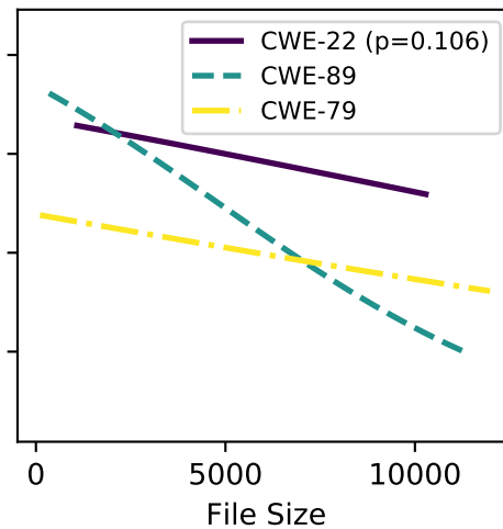
llama-3-70b
