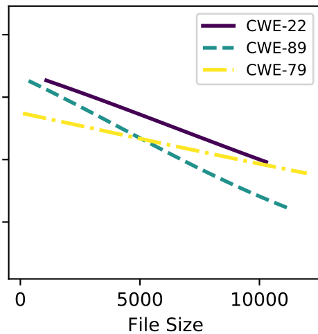
mixtral-8x22b
