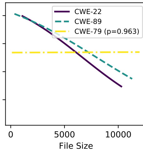
gpt-4-turbo
