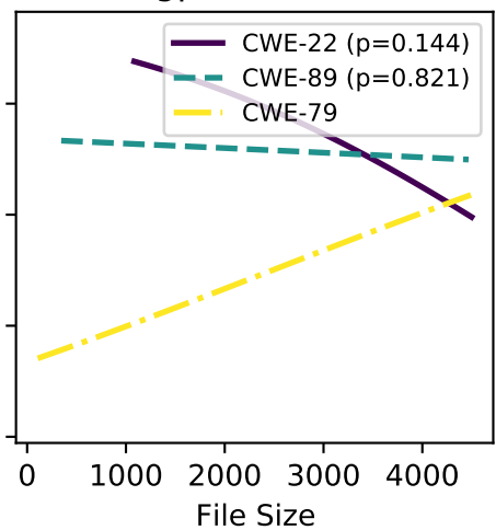
gpt-4-turbo
