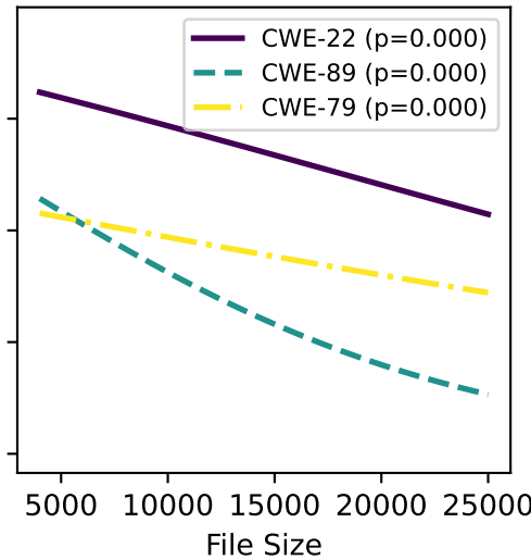
llama-3-70b
