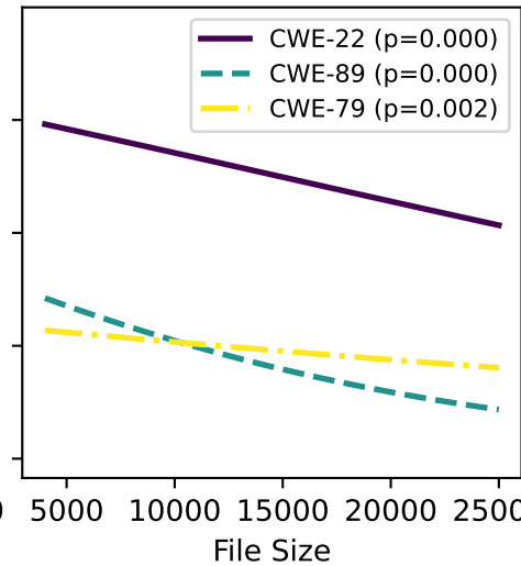
gpt-3.5-turbo
