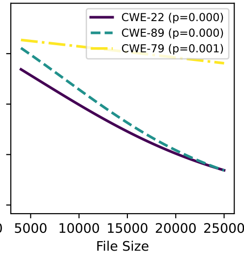
gpt-4-turbo
