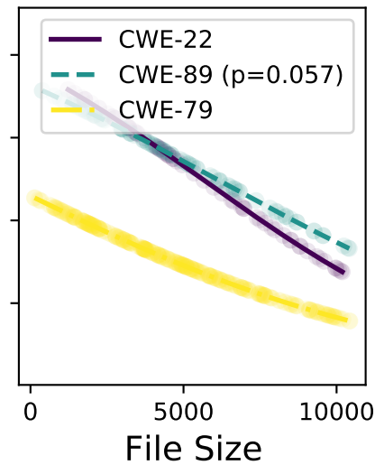
llama-3-70b-8192
