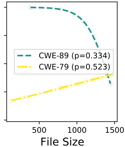
llama-3-70b-8192
