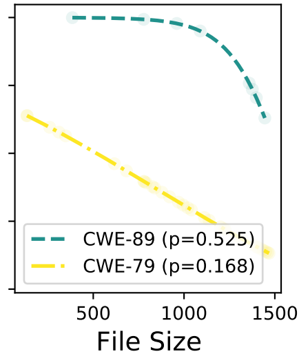
mixtral-8x22b
