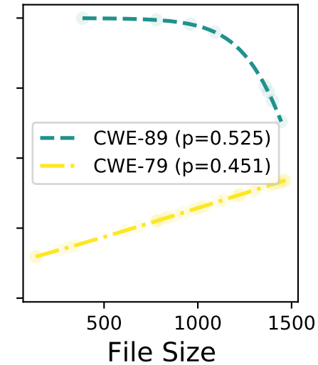
gpt-4o
