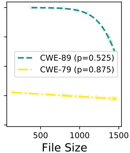
gpt-4-turbo
