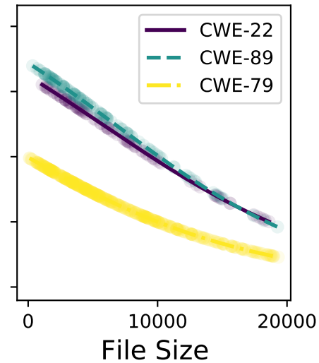
llama-3-70b-8192
