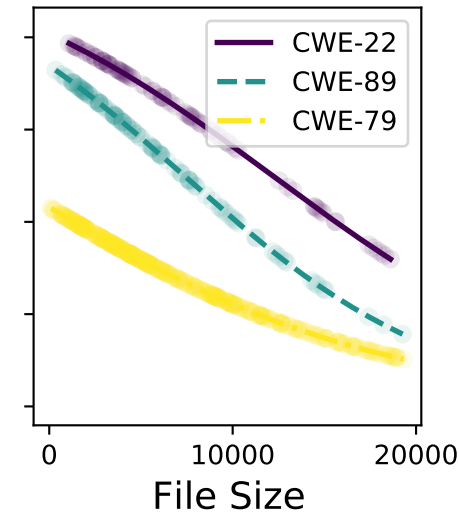
gpt-4-turbo
