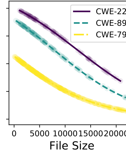
gpt-4-turbo
