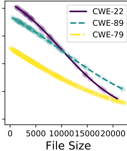
gpt-4o
