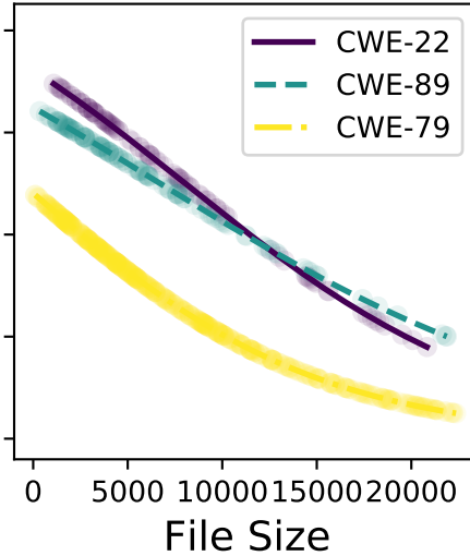
mixtral-8x22b
