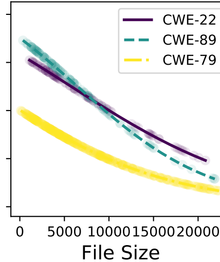
llama-3-70b-8192
