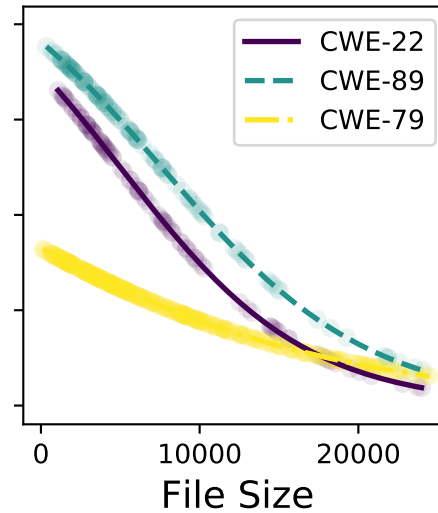
gpt-3.5-turbo
