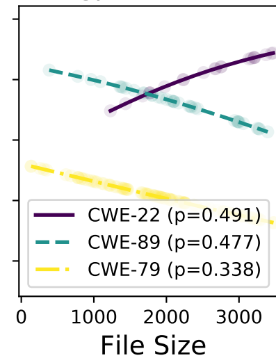
gpt-4-turbo
