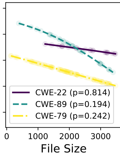
mixtral-8x22b
