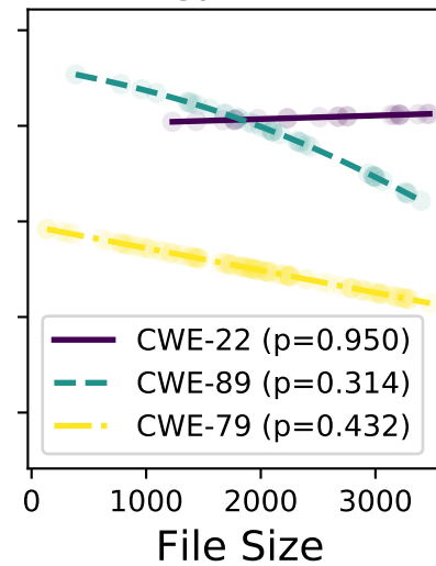
gpt-4o
