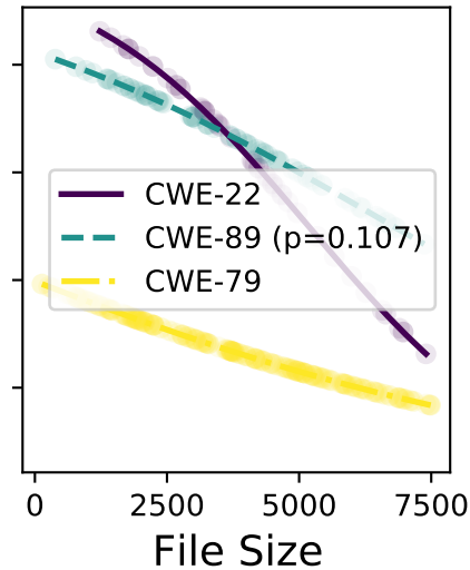
gpt-3.5-turbo
