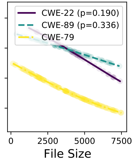
llama-3-70b-8192
