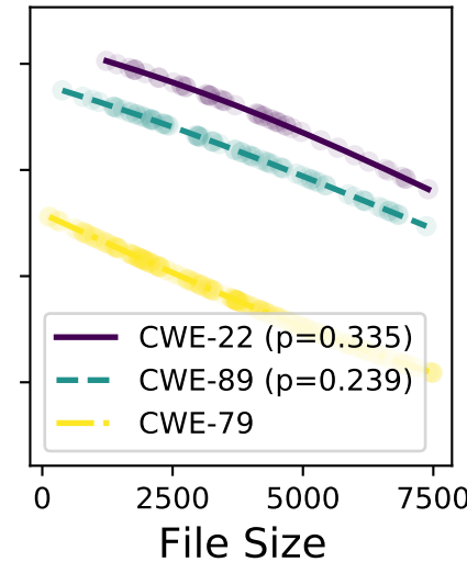
gpt-4-turbo
