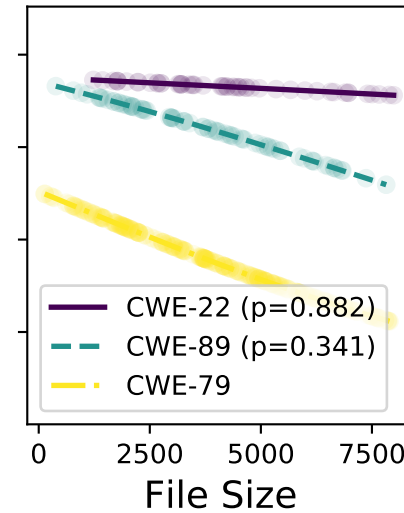
gpt-4-turbo
