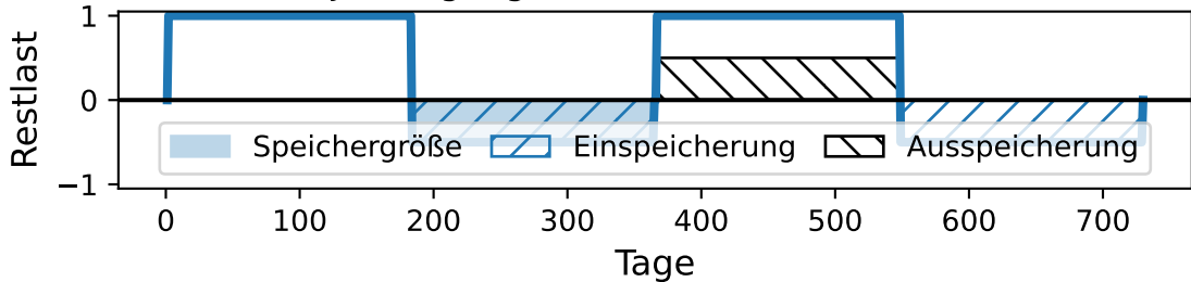
2 Jahressgänge der Restlast bei EE-Defizit
