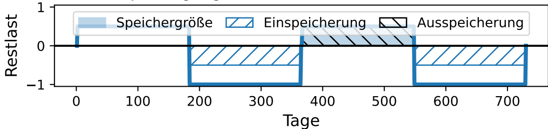
2 Jahressgänge der Restlast bei EE-Überschuss
