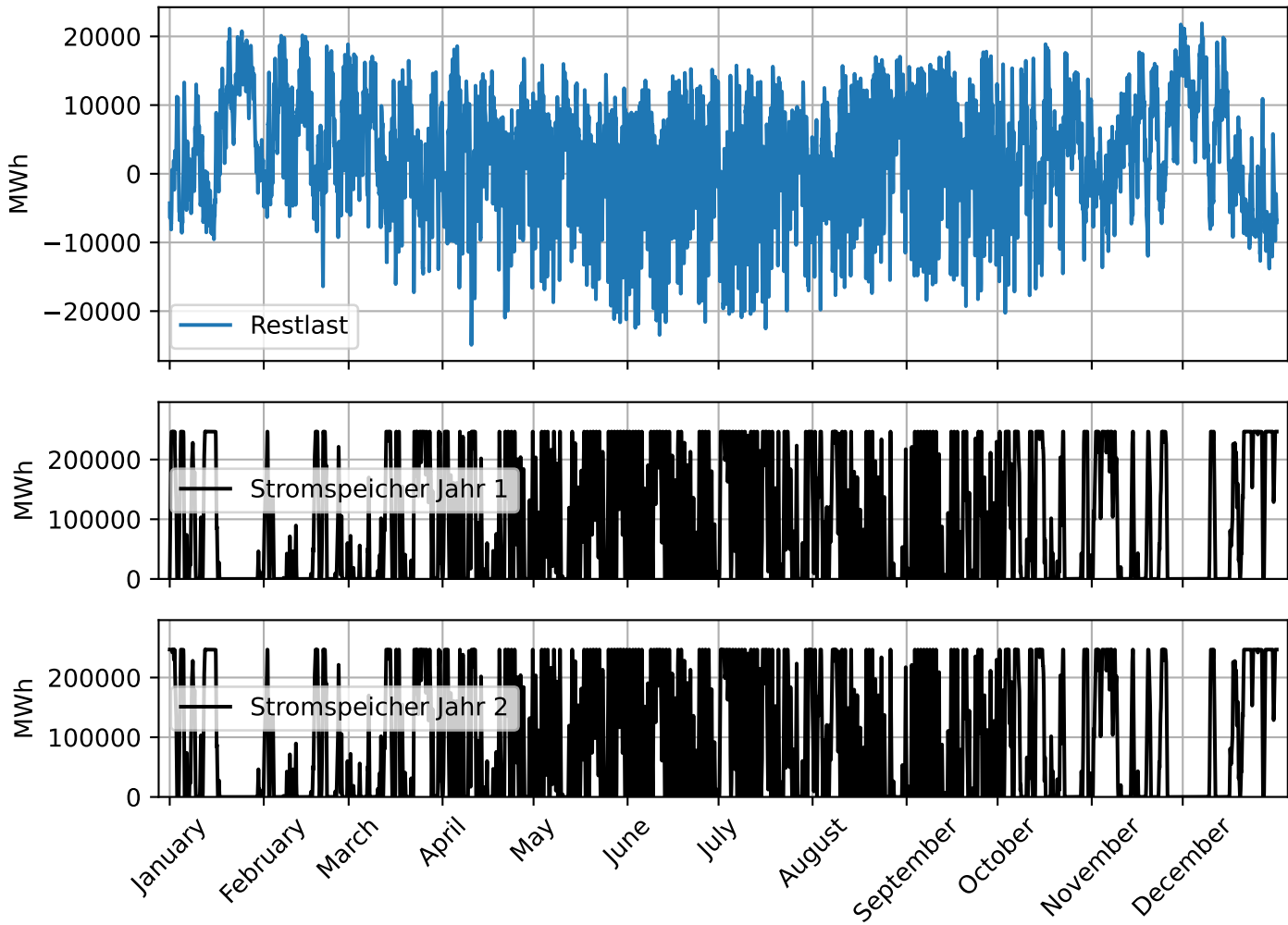
Restlast 2030 und Jahresgang eines Speichers mit C_{max} = 0.04 , \eta_{ein} = 0.9 und \eta_{aus} = 0.88
