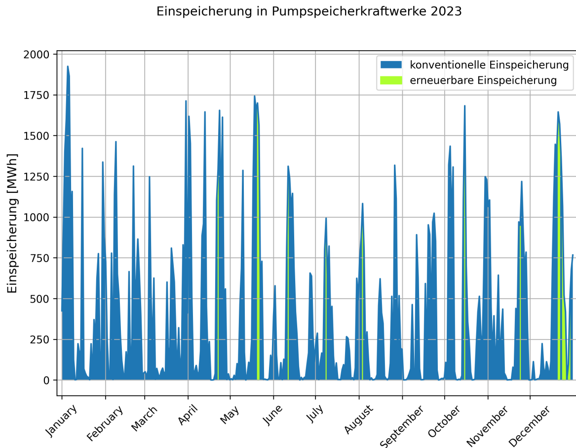
Abbildung 6.11: Einspeicherung in Pumpspeicherkraftwerke 2023
