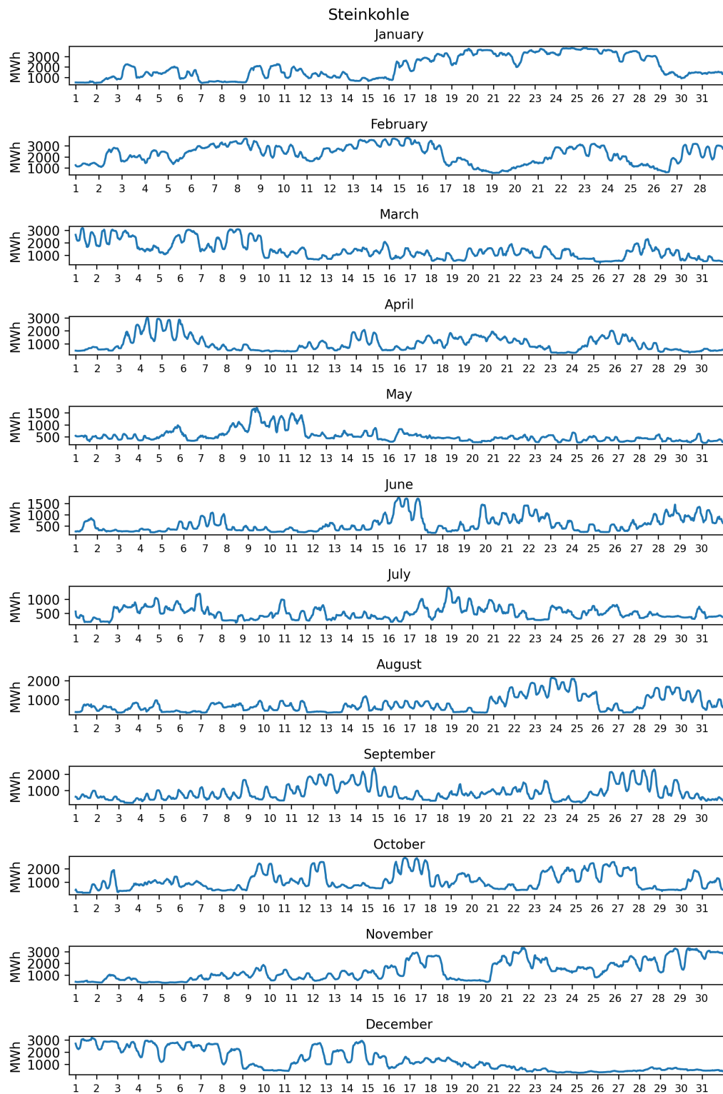
42 Abbildung 6.5: Jahresgang Steinkohle
