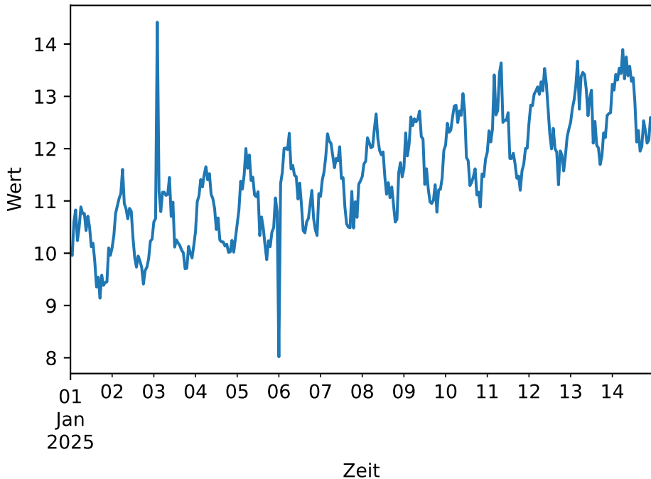
Zeitreihe (Trend + Saison + Rauschen)
