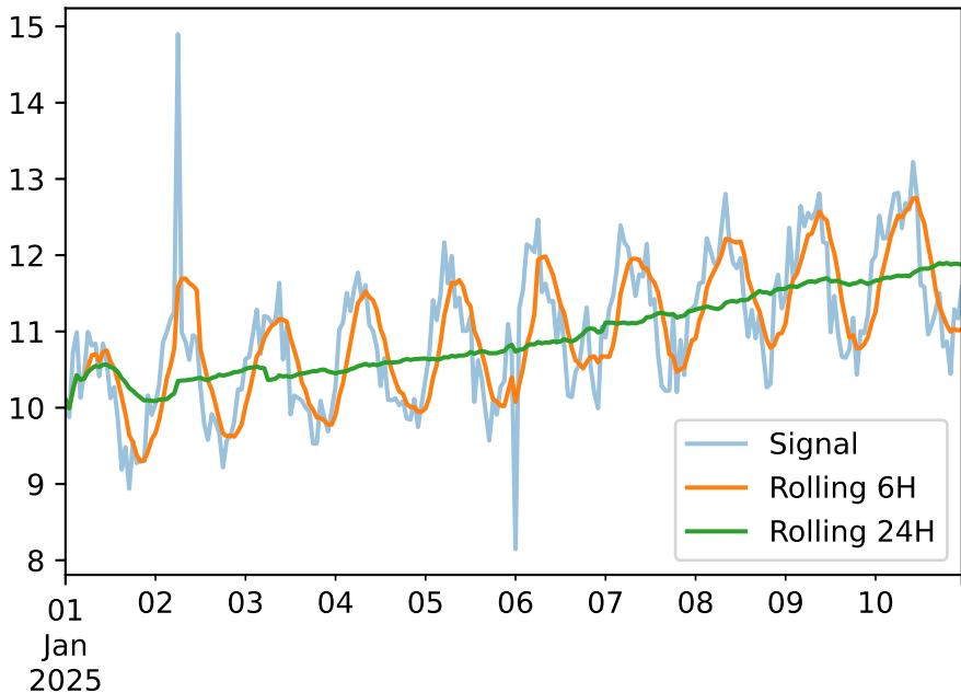
Rolling Mean (Pandas)
