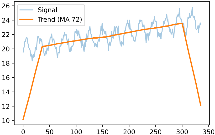
Trend-Schätzung (NumPy)
