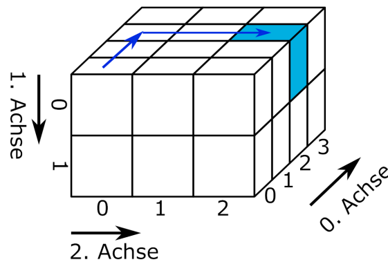
Abbildung 2.4: dreidimensionale Datensätze
