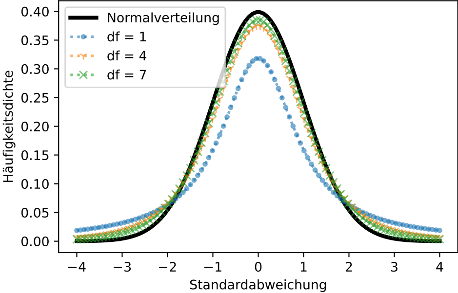
Das Argument df der t-Verteilung
