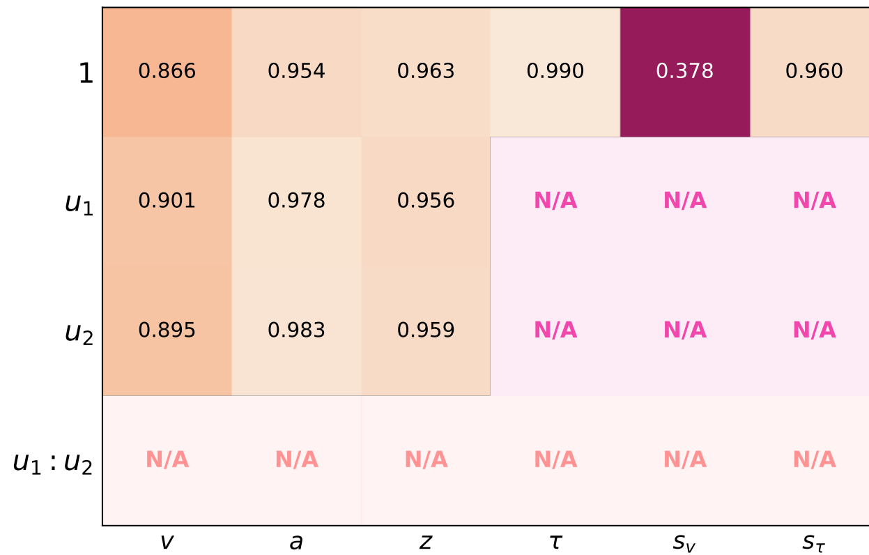
Posterior Contraction
