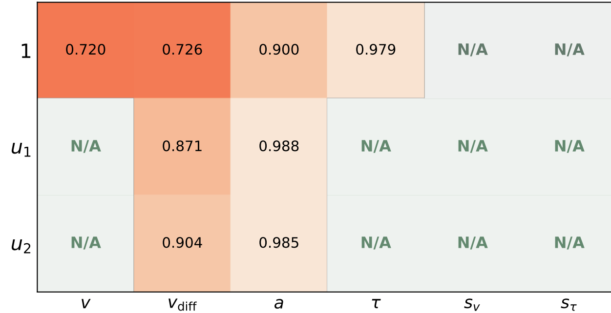
Posterior Contraction
