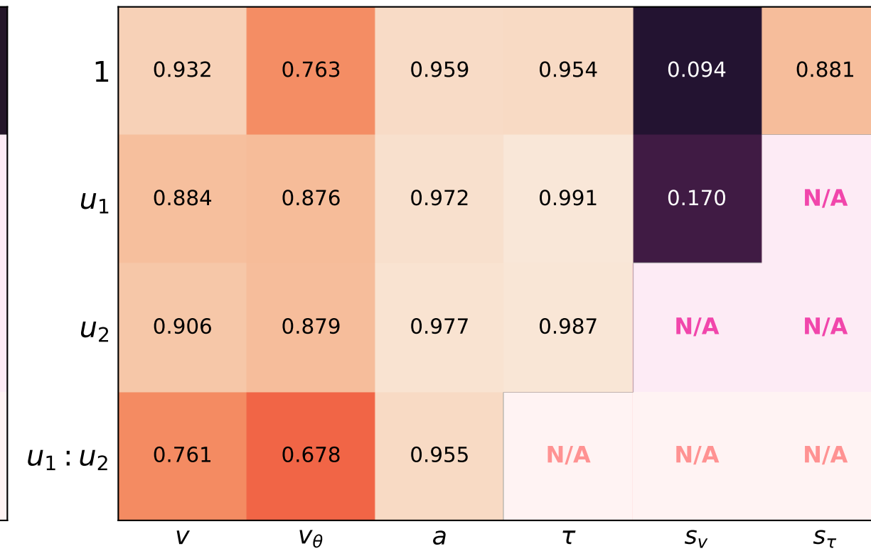
Posterior Contraction
