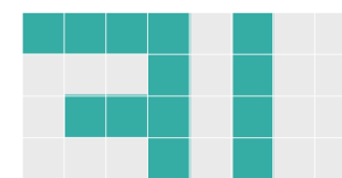
DDM | 2
