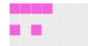
DDM | 5
