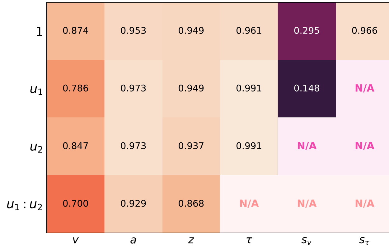
Posterior Contraction
