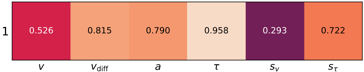
Posterior Contraction
