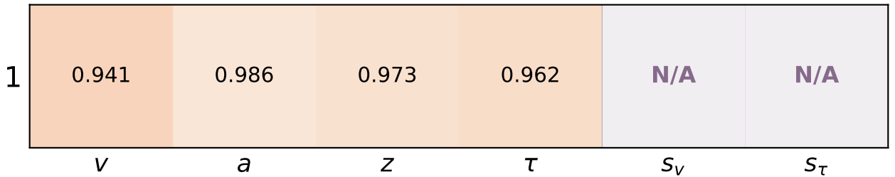
Posterior Contraction
