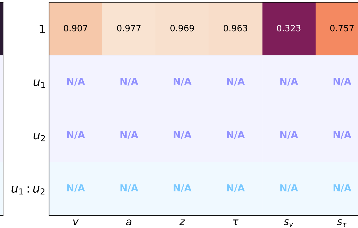
Posterior Contraction
