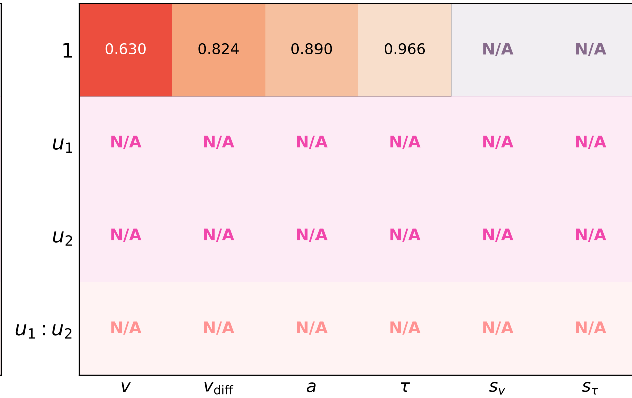
Posterior Contraction
