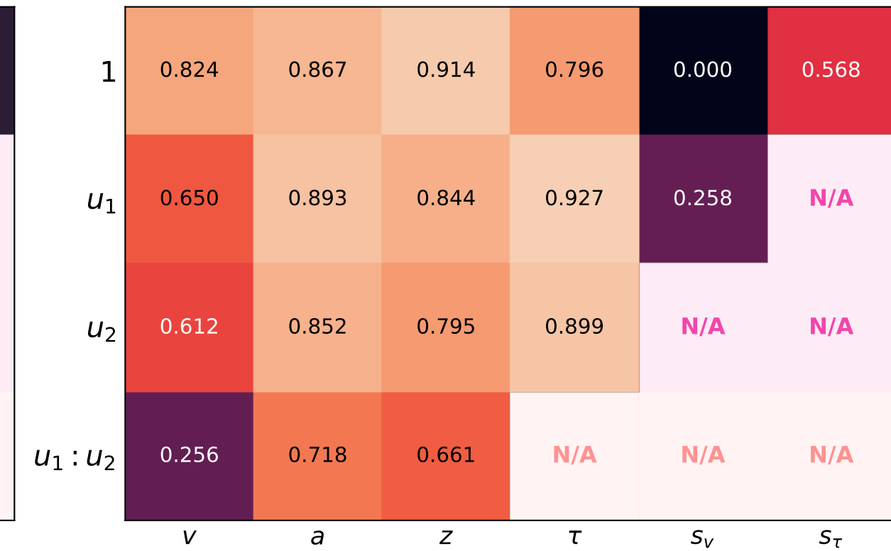
Posterior Contraction
