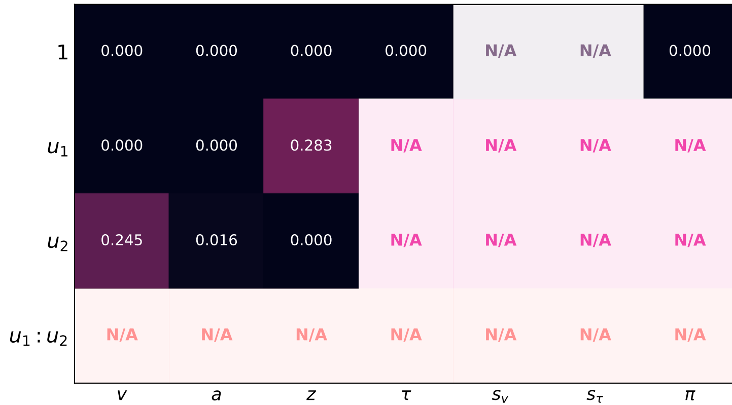
Posterior Contraction
