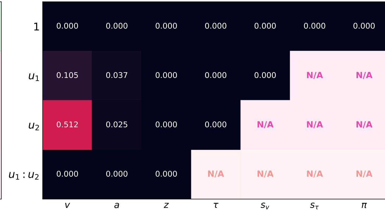
Posterior Contraction
