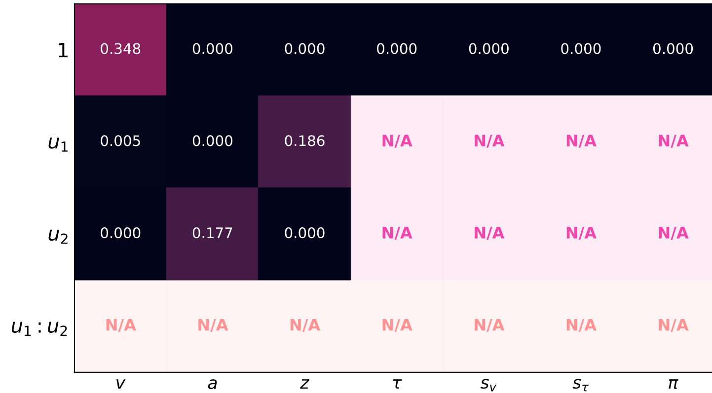
Posterior Contraction
