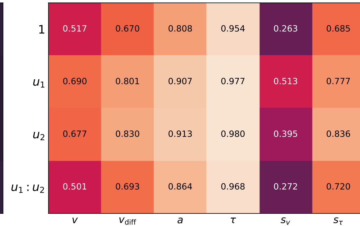
Posterior Contraction
