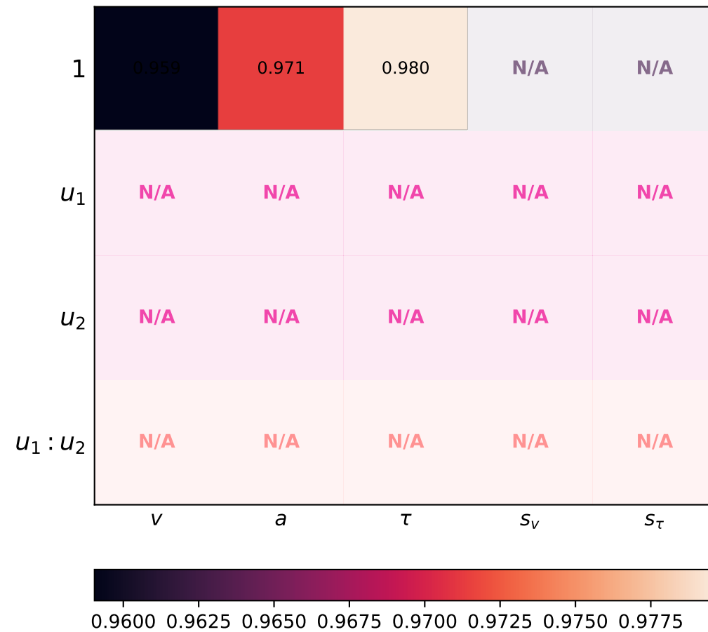
Posterior Contraction
