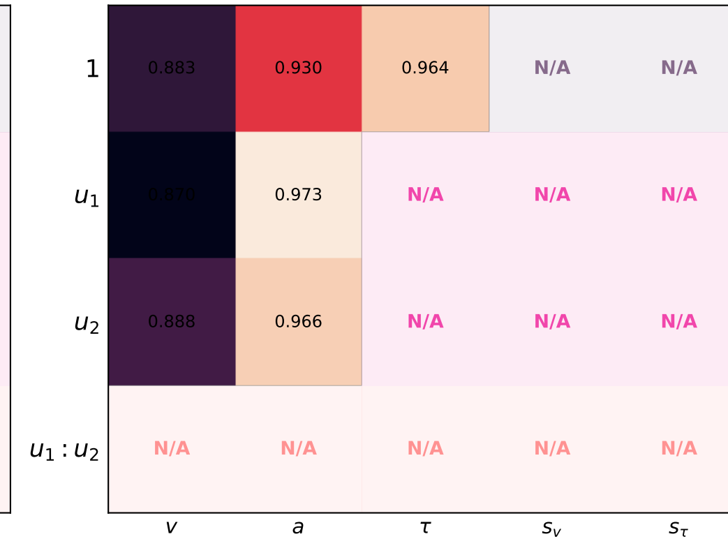
Posterior Contraction
