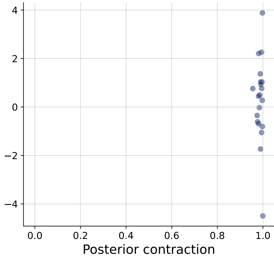
Posterior z-score
