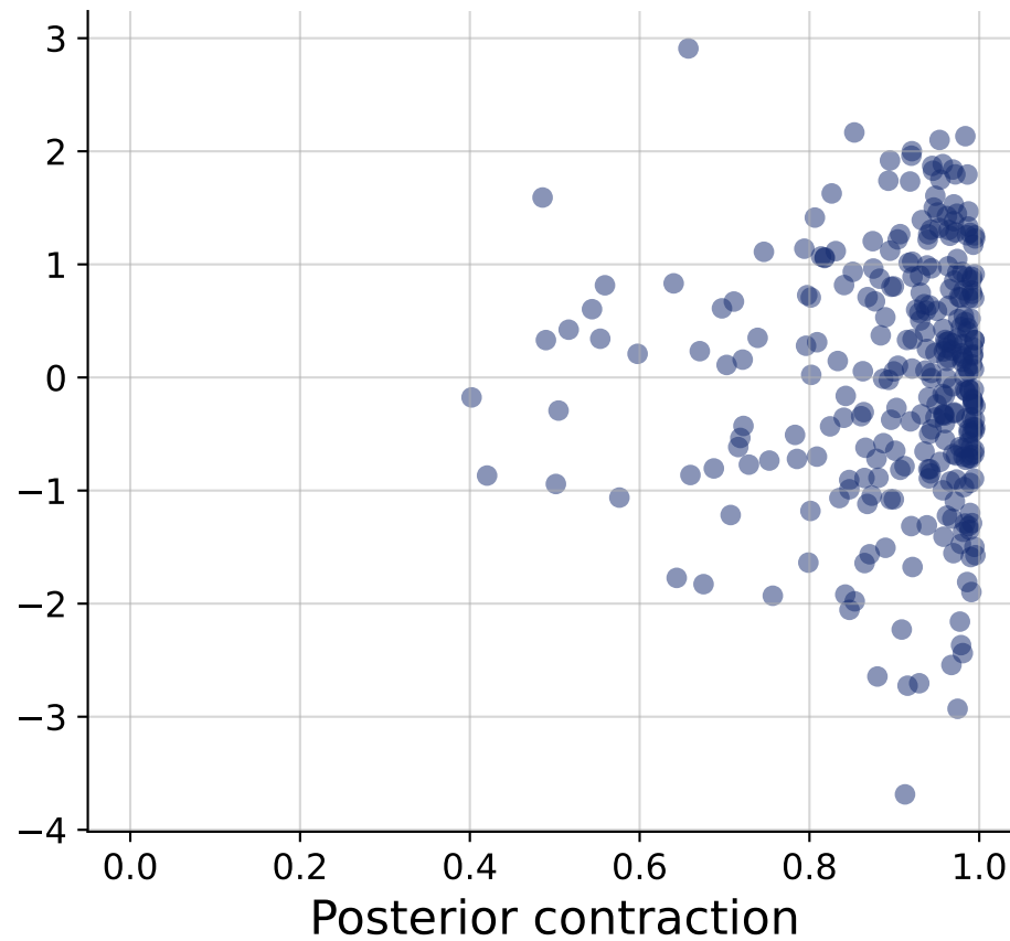
Posterior z-score
