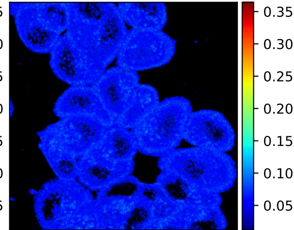
Posterior MAD \tau^{\text{mean}}
