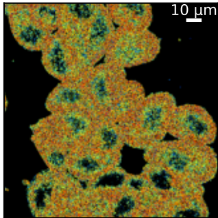
MLE
