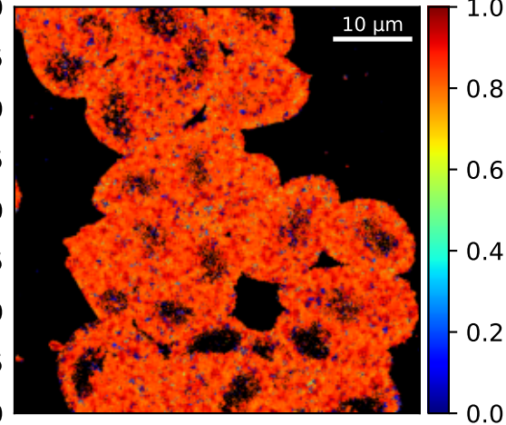
Estimates MLE A^L
