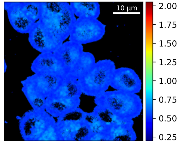
Posterior Median \tau_1^L
