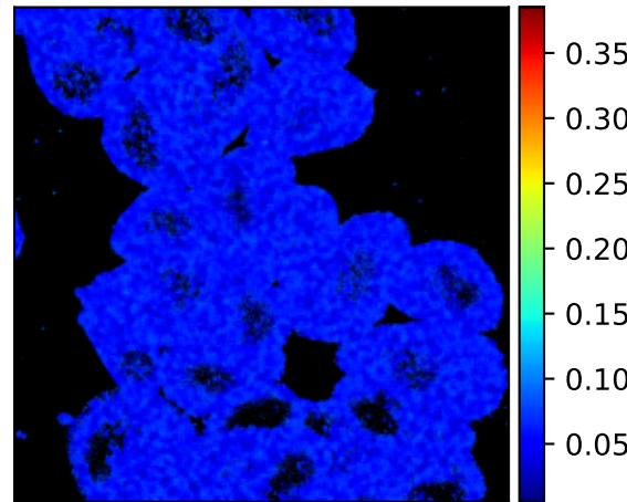
Posterior MAD \tau_2^L
