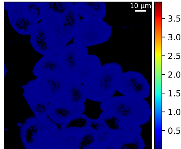
Posterior MAD \tau_1^L
