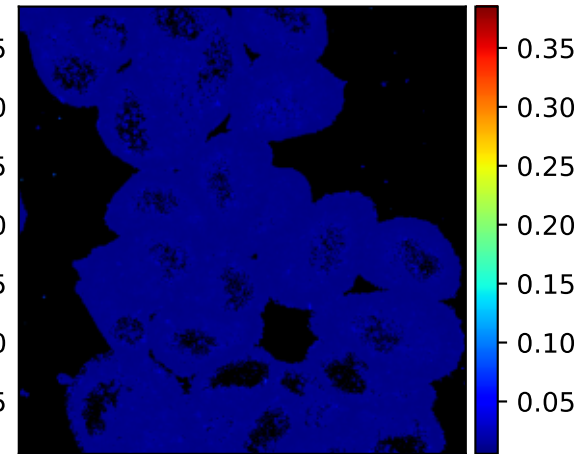
Posterior MAD \tau^{\text{mean}}
