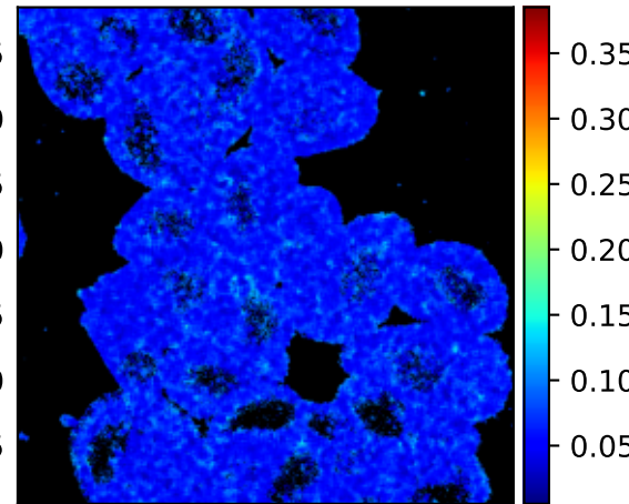
Posterior MAD A^L
