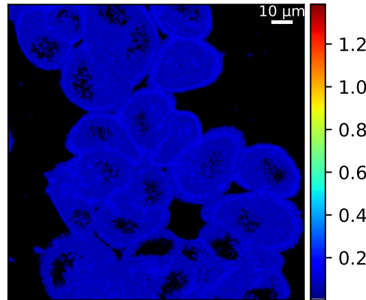
Posterior MAD A^L
