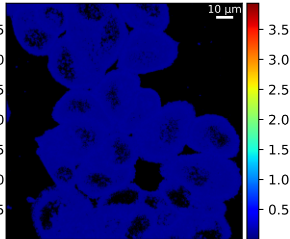
Posterior MAD A^L
