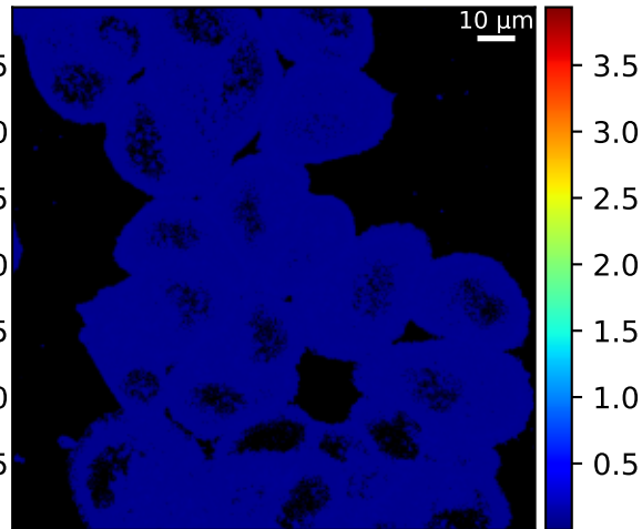
Posterior MAD \tau_2^L
