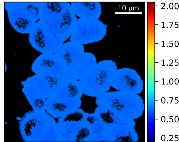
Posterior Median A^L
