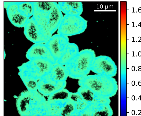
Posterior Median A^L
