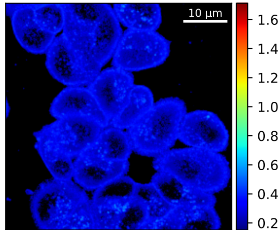
Posterior Median \tau_1^L
