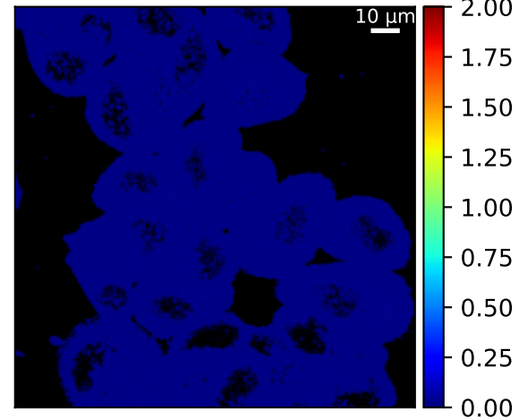
Posterior MAD \tau^{\text{mean}}
