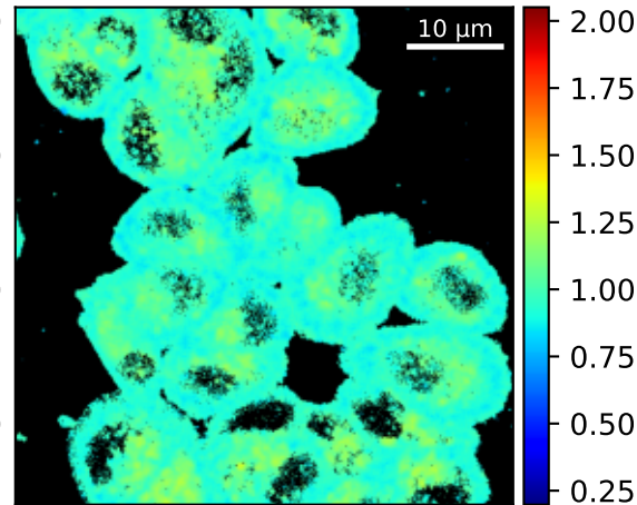
Posterior Median \tau^{\text{mean}}
