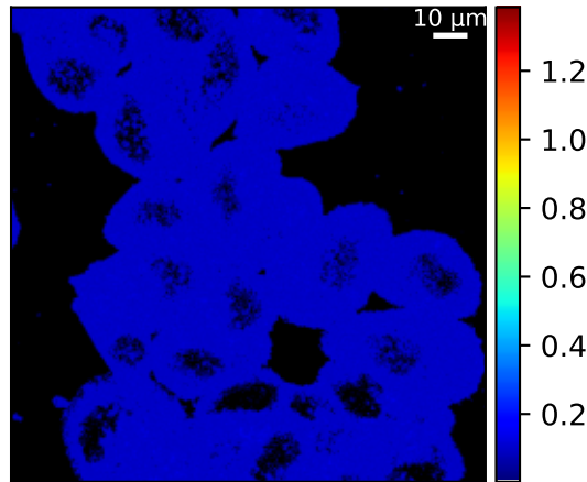
Posterior MAD \tau_2^L
