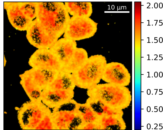
Posterior Median \tau_2^L
