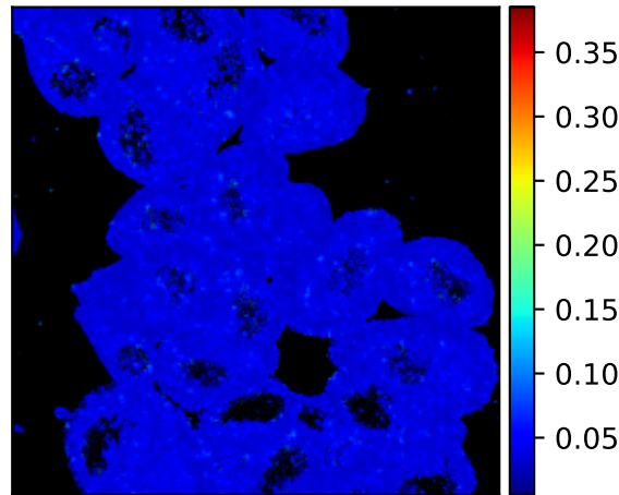
Posterior MAD \tau_1^L
