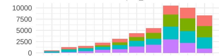
cathepsin_B
