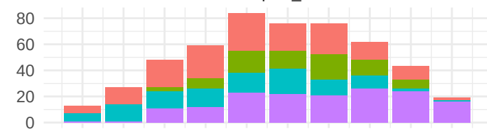
cathepsin_D
