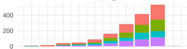
cathepsin_B
