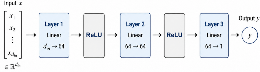
그림 3: 비용 신경망 하나의 구조. 입력은 후보 하나에 대한 고정 길이 특징 벡터이고 두 개의 64차원 은닉층에는 ReLU 활성화함수를 적용한다. 출력은 그 후보의 짝 중심 비용 점수 하나다. 한 번의 결정은 같은 망으로 후보를 각각 평가한 뒤 \arg \min 을 취한다. 제안 정책과 수락 정책은 이 구조를 공유하며 입력 차원만 각각 21과 16으로 다르다.
