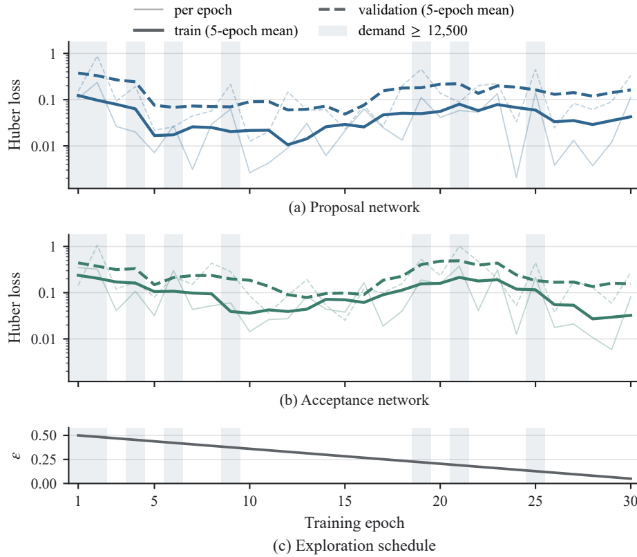
그림 7: 30회차 동안의 학습·검증 손실. 회차별 원값을 열게 깔고 그 위에 다섯 회차 이동평균을 얹었다. (a) 제안망과 (b) 수락망은 서로 다른 결정으로 적합하므로 따로 그렸고, 손실이 세 자릿수를 오가므로 세로축은 로그다. (c) 탐색 확률 \varepsilon 은 0.50에서 0.05로 선형 감소한다. 음영은 그 회차에 뽑힌 수요가 하루 12,500대 이상이었음을 뜻한다. 수요를 회차마다 새로 뽑기 때문에 17-24회차의 상승을 포함해 눈에 보이는 출렁임의 상당 부분은 적합이 아니라 그 추첨을 따른다.
