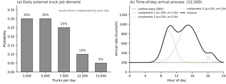
Fig. 2: 외부 트럭 작업 수요. (a) 다섯 개의 일일 수요 수준과 각각이 뽑힐 확률이며 날마다 독립으로 추첨한다. (b) 혼잡 수준 하나에서의 도착 과정으로, 균등 기저와 가우시안 성분셋을 따로 그렸다. 선행연구가 뒷받침하는 것은 수요 규모와 도착이 하루 중 균일하지 않다는 사실이고, 혼합의 형태는 본 연구의 구성이다.
