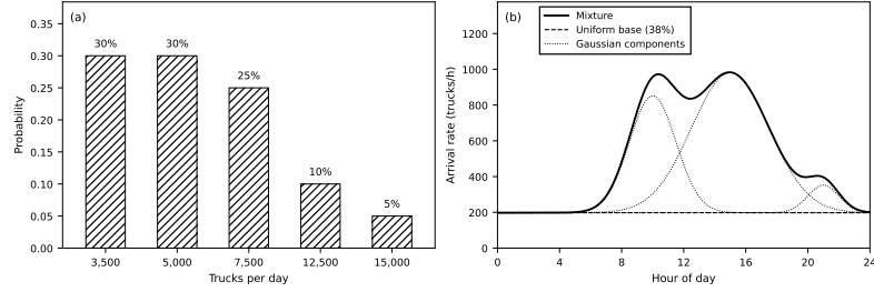
Fig. 2: 외부 트럭 작업 수요. (a) 다섯 개의 일일 수요 수준과 각각이 뽑힐 확률이며 날마다 독립으로 추정한다. (b) 하루 12,500대 조건의 시간대별 도착 과정으로, 균등 기저와 가우시안 성분 셋을 이들이 합쳐 이루는 곡선 아래에 따로 그렸다. 선행연구가 뒷받침하는 것은 수요 규모와 도착이 하루 중 균일하지 않다는 사실이고, 혼합의 형태는 본 연구의 구성이다.
