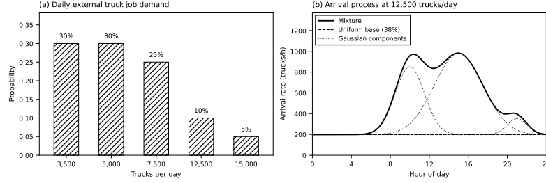
Fig. 2: 외부 트럭 작업 수요. (a) 다섯 개의 일일 수요 수준과 각각이 뽑힐 확률이며 날마다 독립으로 추첨한다. (b) 혼합 수준 하나에서의 도착 과정으로, 균등 기저와 가우시안 성분 셋을 따로 그렸다. 선행연구가 뒷받침하는 것은 수요 규모와 도착이 하루 중 균일하지 않다는 사실이고, 혼합의 형태는 본 연구의 구성이다.
