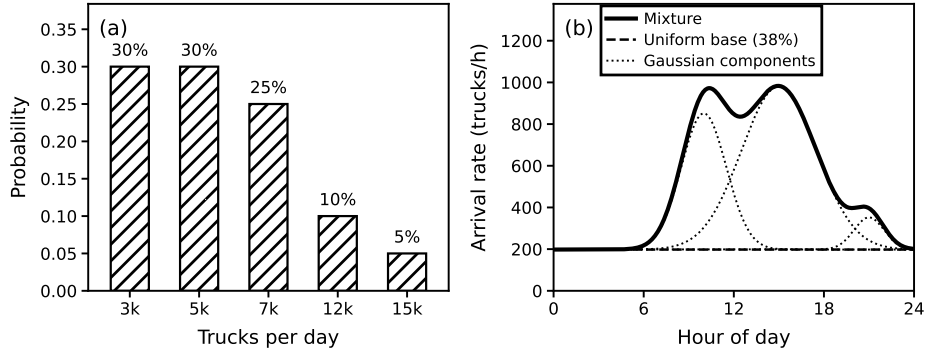
Fig. 2: 외부 트럭 작업 수요. (a) 다섯 개의 일일 수요 수준과 각각이 뽑힐 확률이며 날마다 독립으로 추정한다. (b) 하루 12,500대 조건의 시간대별 도착 과정으로, 균등 기저와 가우시안 성분 셋을 이들이 합쳐 이루는 곡선 아래에 따로 그렸다. 선행연구가 뒷받침하는 것은 수요 규모와 도착이 하루 중 균일하지 않다는 사실이고, 혼합의 형태는 본 연구의 구성이다.
