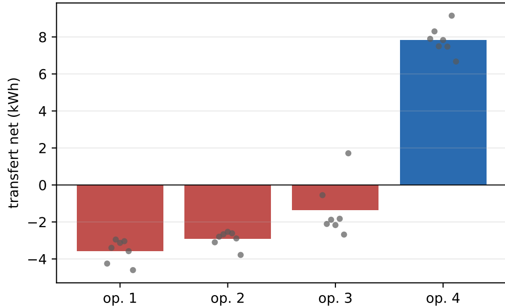
(b) \tau_i Shapley : négatif = paie
