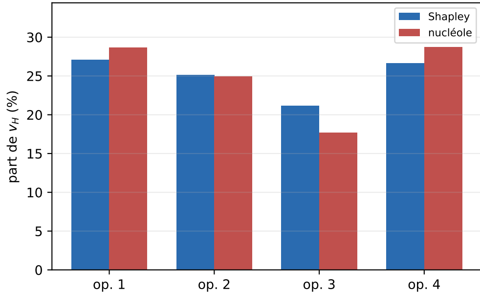
(a) répartition des économies, moyenne des 7 nuits
