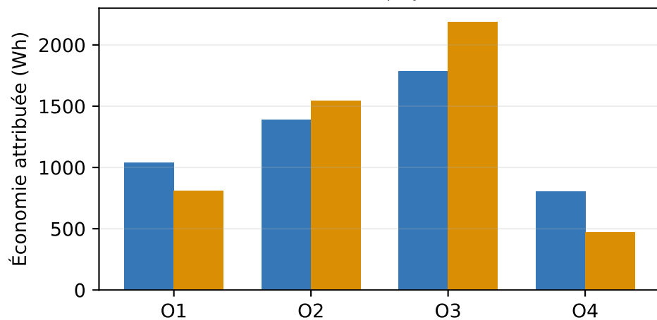
Cœur non vide, Shapley hors du cœur
