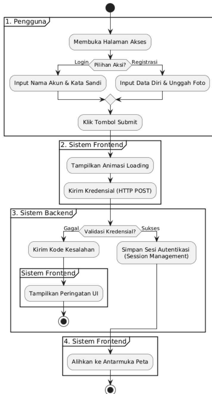
Gambar 3.2 Activity Diagram Manajemen Autentifikasi dan Profil
