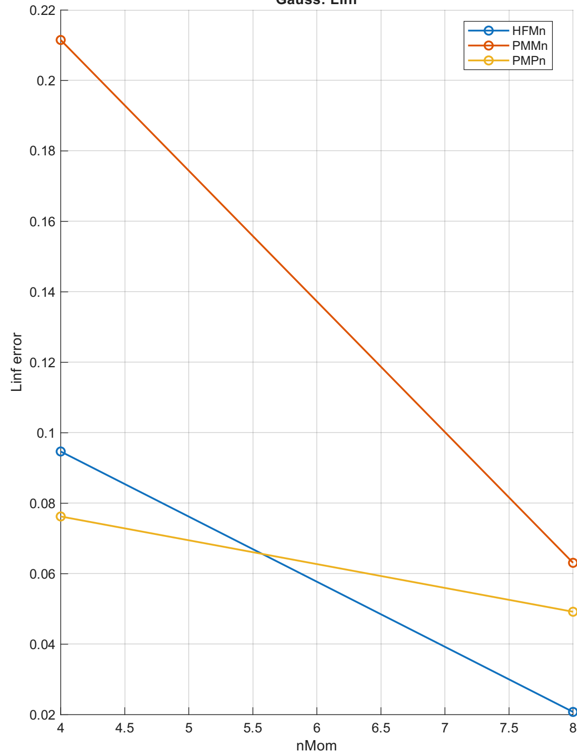
Gauss: Linf
