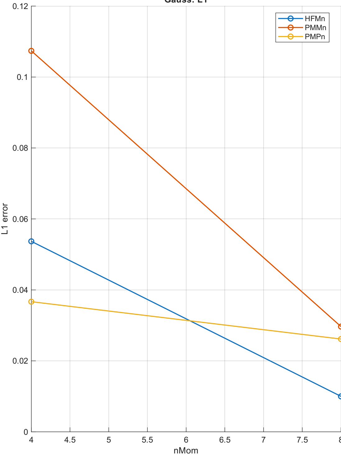
Gauss: L1
