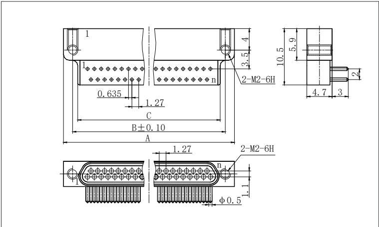
J30JZLN □ ZKWA000（9、15、21、25、31、37 芯）
